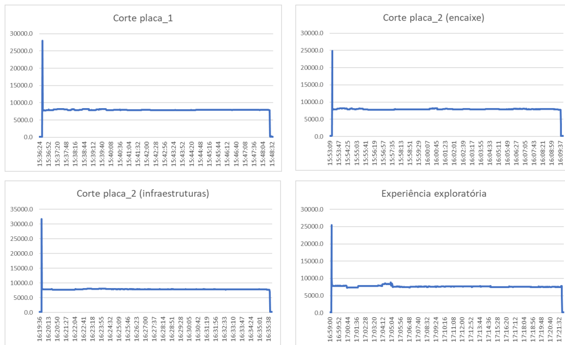
Figura 166. CNC – Gráficos de consumo.
