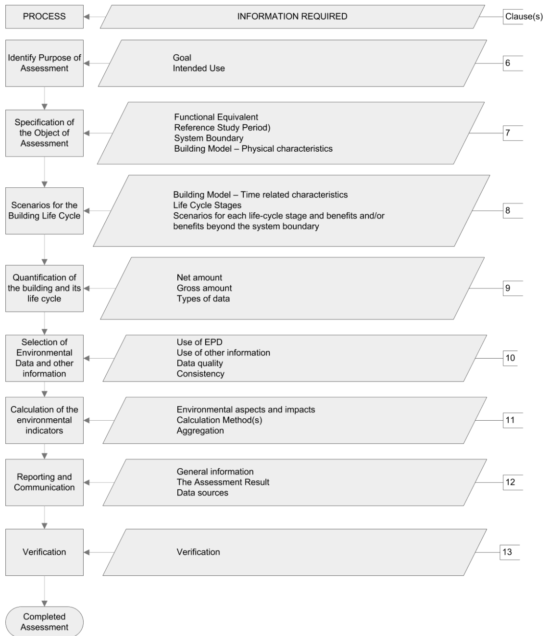
Figura 3. Fluxograma do processo de avaliação do desempenho ambiental do edifício.
