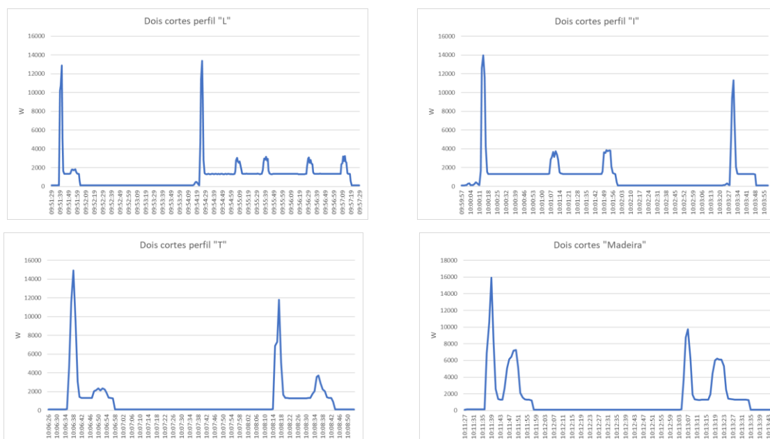
Figura 133. Máquina de Corte – Consumo.
