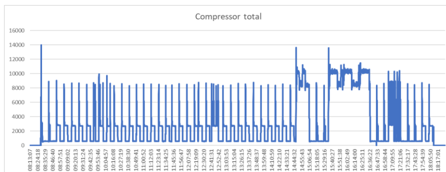
Figura 122. Compressor – Consumo.
